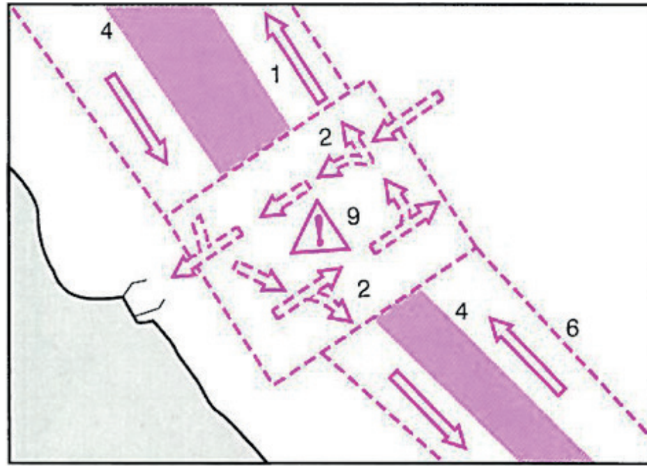
Figure 8 Zone de prudence au niveau d'une jonction avec des sens recommandés de flux de circulation
