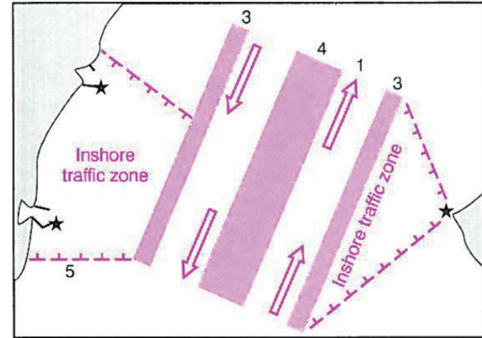
Figure 6 Zones de navigation côtière
