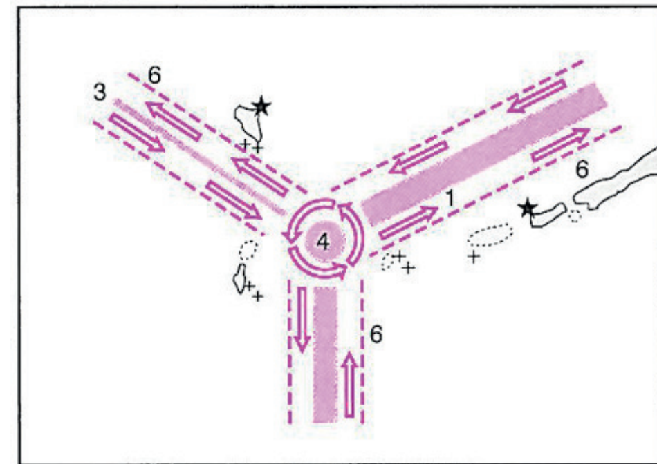
Figure 11 Séparation du trafic au niveau d'un rond-point
