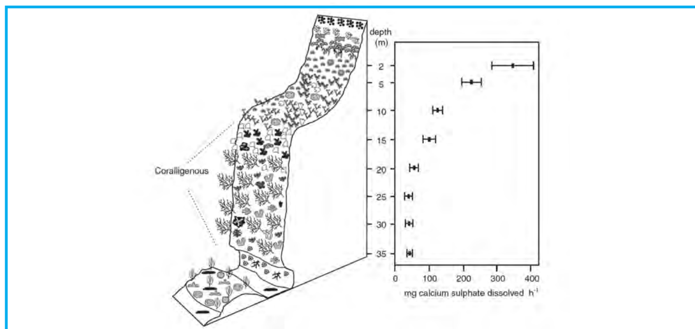
Figure 8. Moyenne annuelle de l'atténuation du mouvement de l'eau (moyenne \pm écart type) pour une profondeur entre 0 et 35 m dans un mur sous-marin aux îles Medes. (Redessiné d'après Garrabou, 1997).
