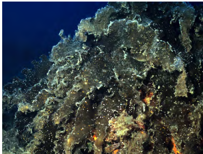
Figure 151. Des bancs de varech de Laminaria rodriguezii , endémiques et menacés, remplacent les affleurements coralligènes près des événements de CO 2 des îles Columbretes (Espagne), à -40 m de profondeur (Photo de E. Ballesteros).
