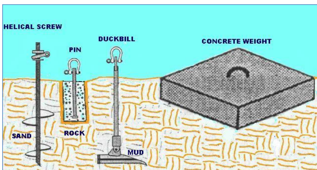
Figura 2. Bllloqe të mëdha betoni që dëmtojnë zona të mëdha të fundit të detit, nuk rekomandohen më për vendet ku gjenden livadhet detarë Posidonia. Në varësi të natyrës së detit, vidhat spirale, kunjat e ankoruara ne plinta betoni ose spiranca “sqep-rose” tani janë të detyrueshme në zonat ku ndalohet ankorimi
