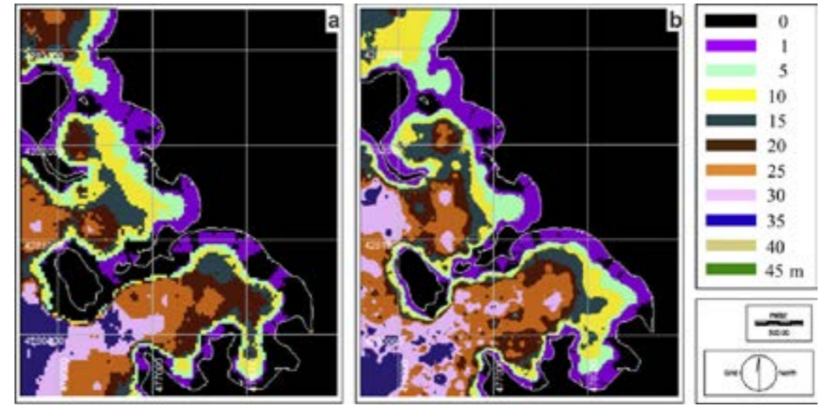
Şekil 8 (a) Aster, (b) Quickbird ANN modelleri ile oluşturulan batimetri haritaları (Kaynak: Özçelik ve Arısoy, 2010)
