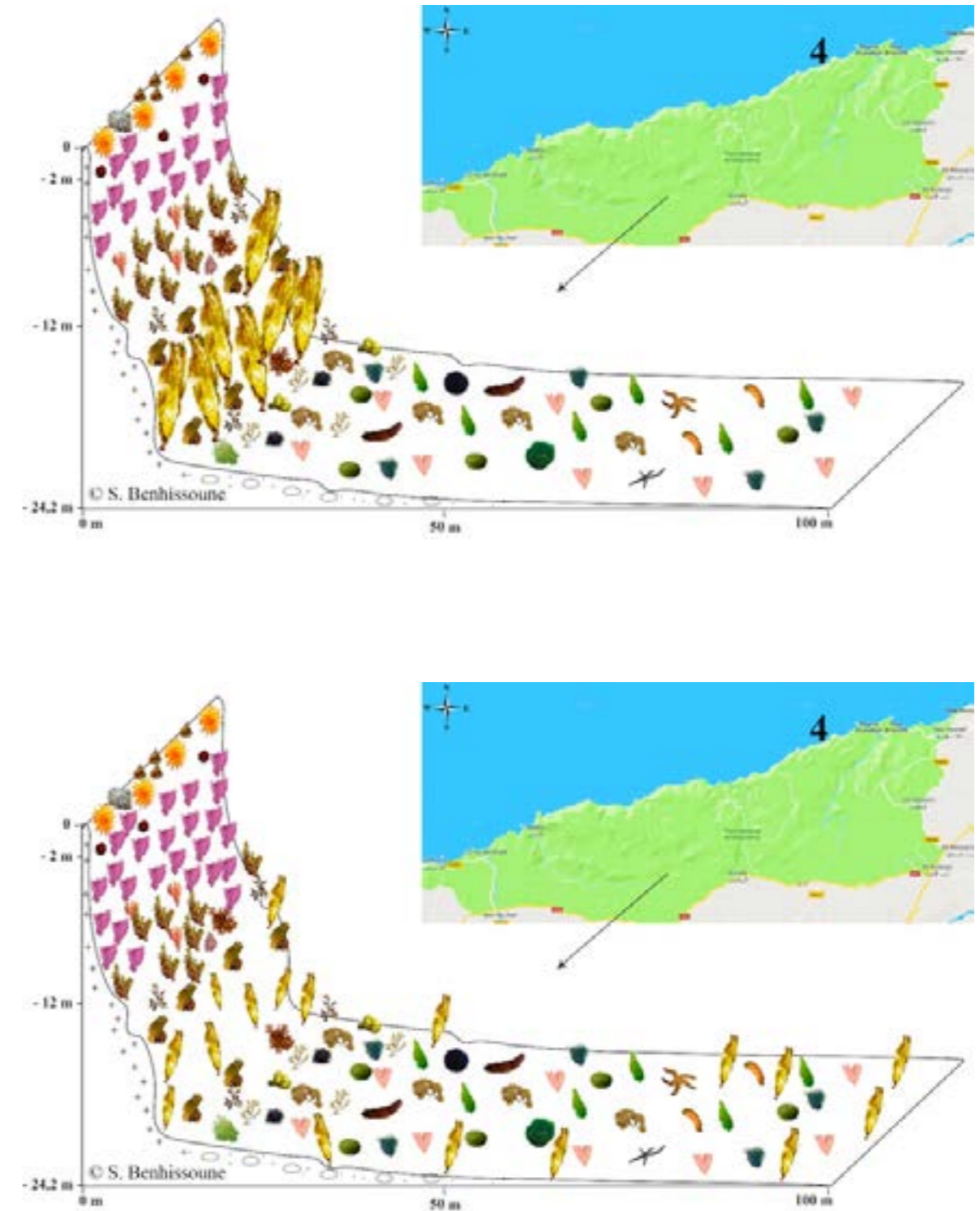
Figure 13 Bloc diagramme synthétique du peuplement benthique au niveau du transect 4 en 2002 (en haut) en 2019 (en bas).
